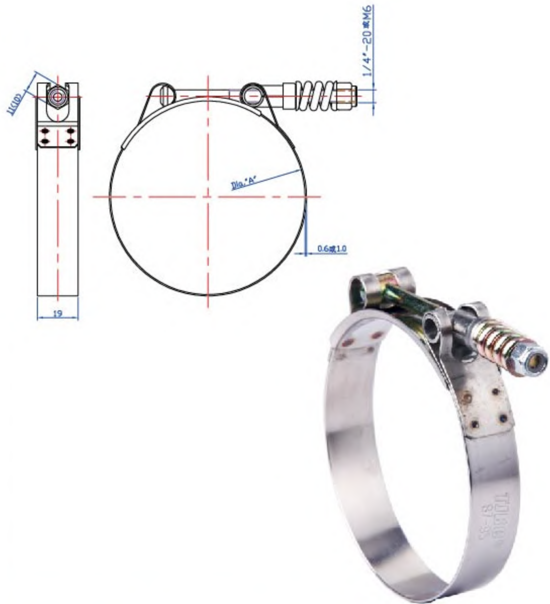
■ QL02 T型弹簧卡箍（T-bolt with spring clamp）
